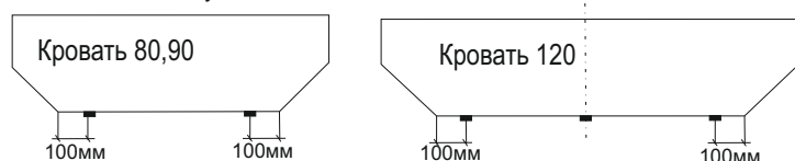
Схема установки подпятников
